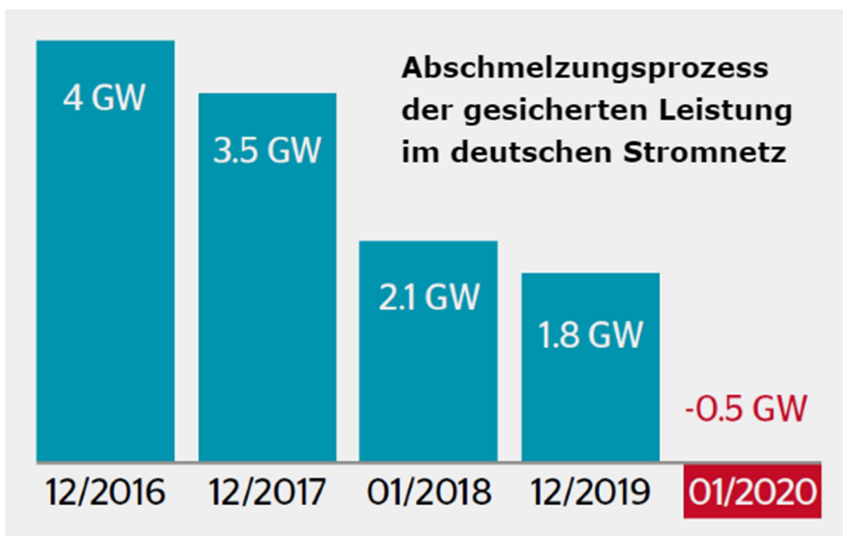
GRAFIK 1 – Abschmelzungsprozess der gesicherten Leistung im deutschen Stromnetz: Bereits vor der Stilllegung der letzten Kernkraftwerksblöcke bis Ende 2022 (= 8 GW) kann sich Deutschland bei kalten Dunkelflauten nicht mehr selbst versorgen. Da die Leistungsknappheit auch in Nachbarstaaten nahezu zeitgleich auftritt, können weitere erzwungene Kraftwerksstilllegungen die Versorgungssicherheit zusätzlich gefährden. Quelle: Bericht zur Leistungsbilanz 2017, 4 ÜNB, Januar 2018
